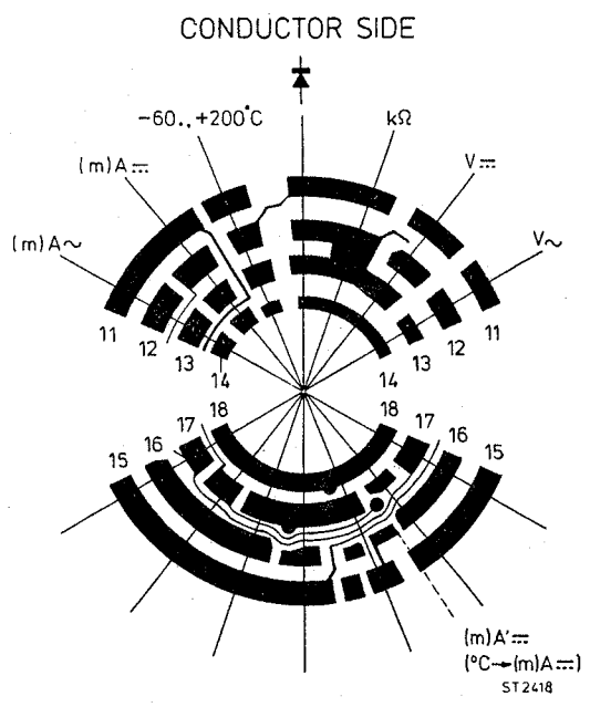
Fig. 52. Function switch lay-out
